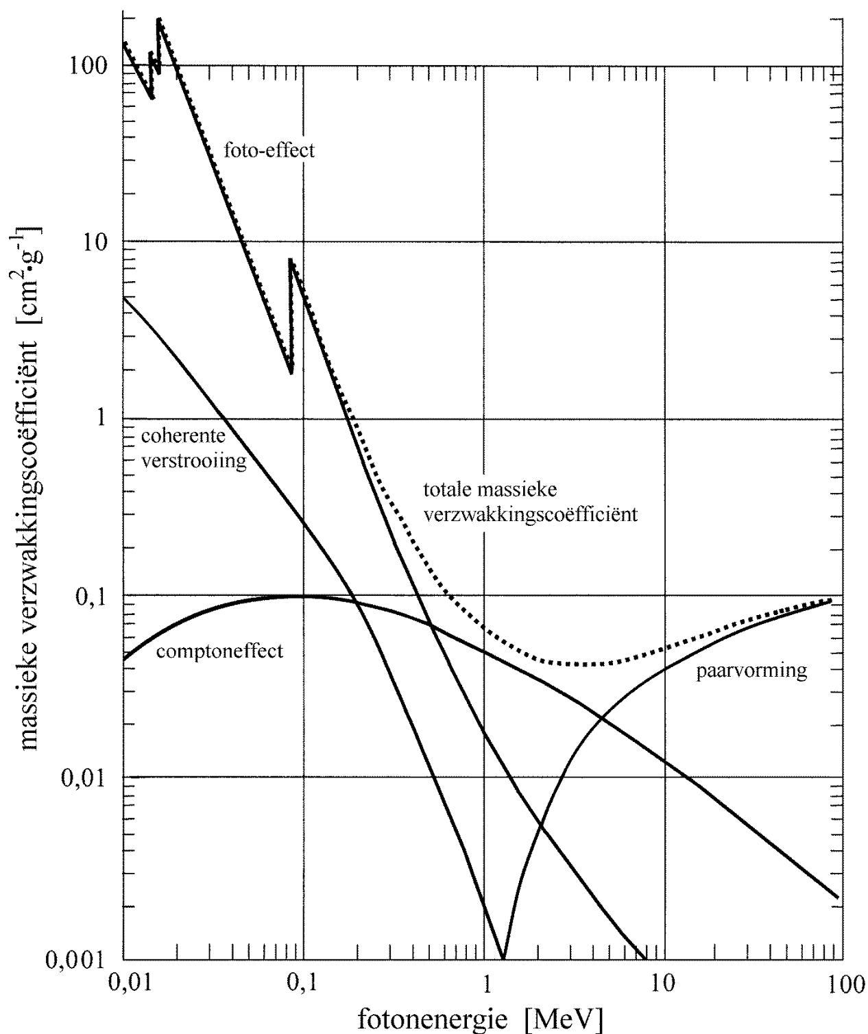
De massieke verzwakkingscoëfficiënt van lood als functie van de fotonenergie
