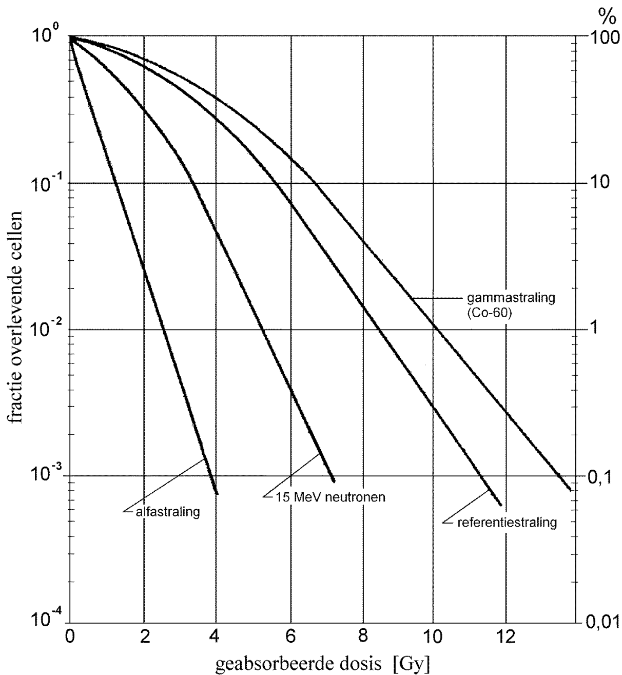
Celoverlevingscurven van alfastraling, van 15 MeV neutronenstraling en van gammastraling van 60 Co
